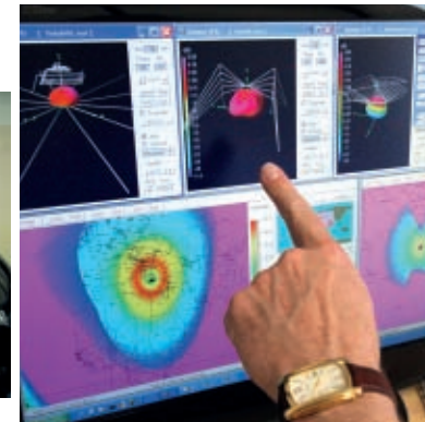
Simulation d'environnement électromagnétique
